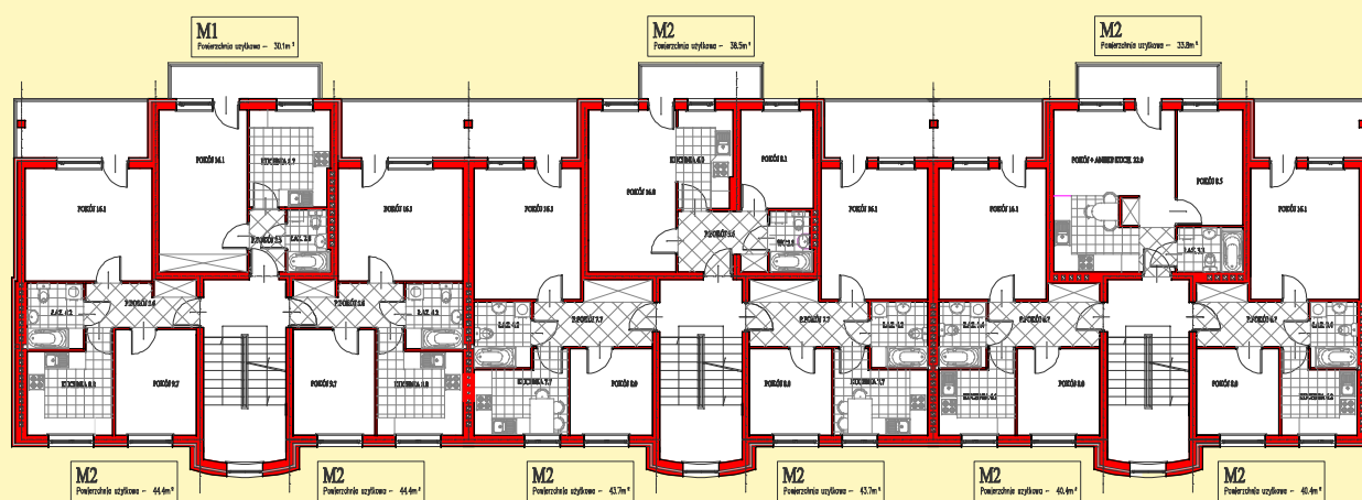
RZUT KONDYGNACJI POWTARZALNEJ
